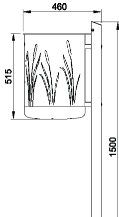
7039-60 Seitenansicht
