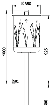
7039-60 Frontansicht
